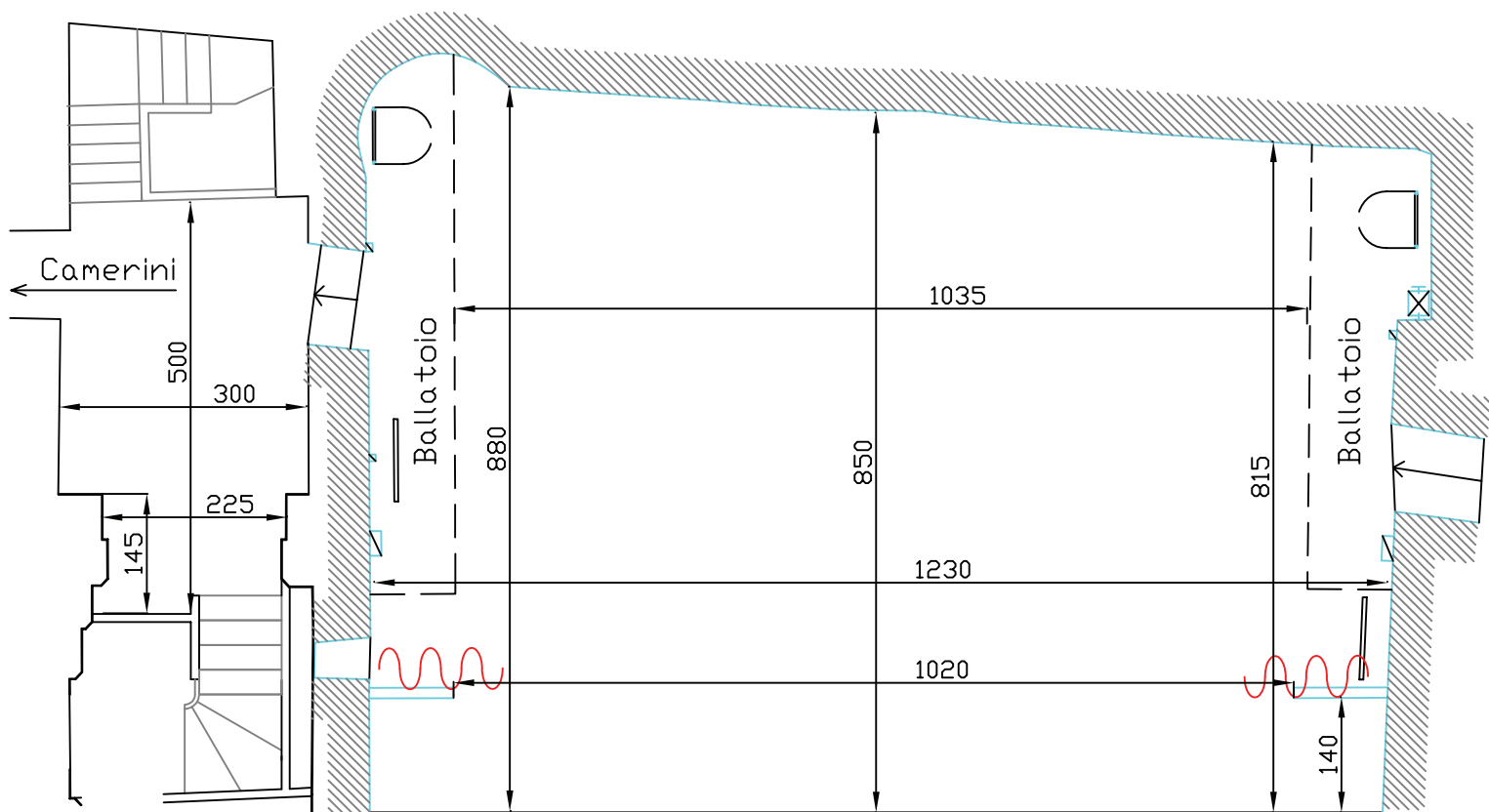
Planimetria palcoscenico Sala Umberto Roma - Declivio 2,75%
